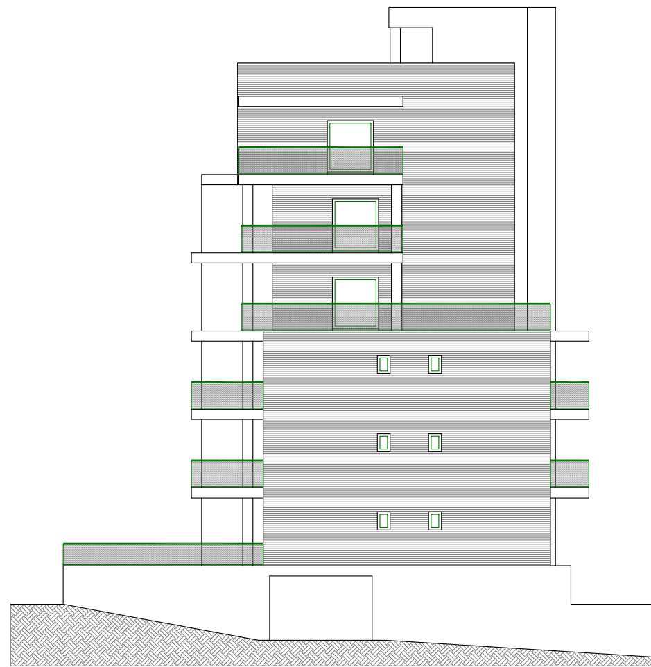
ALZADO OESTE
